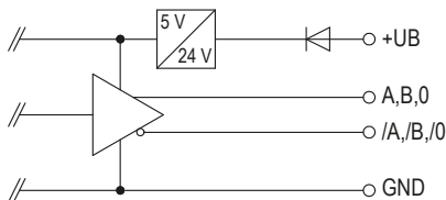
Abb. 3: Ausgangsschaltung LD24
