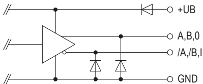
Abb. 5: Ausgangsschaltung OP, ON
