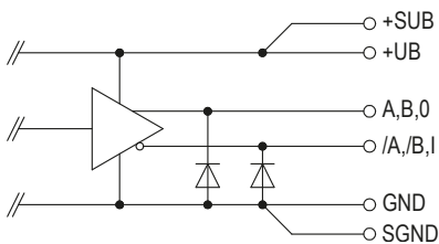
Abb. 7: Ausgangsschaltung LD
