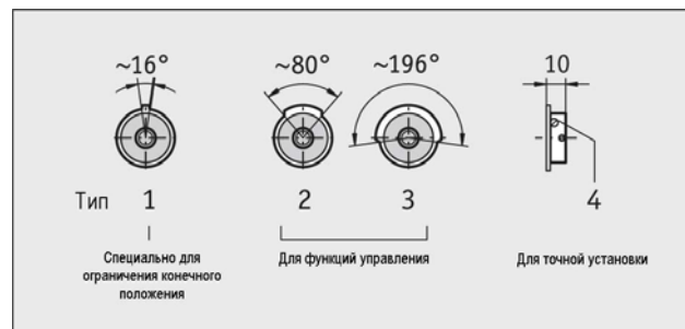
Углы срабатывания для кулачковых переключателей
